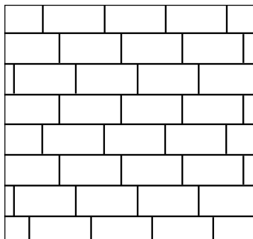
LØPENDE FORBAND Kvart stein
