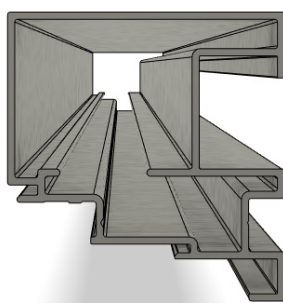
Dækprofil
