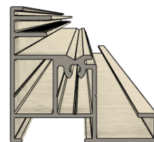
Guide profil till stödben (ZipX95)
